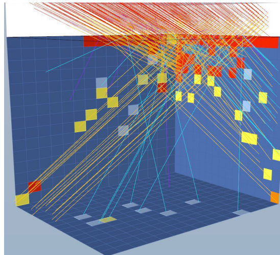
COMPARAISON DES RAYONS RÉFLÉCHIS AVANT ET APRÈS LA CONSTRUCTION DE LA VERRIÈRE
