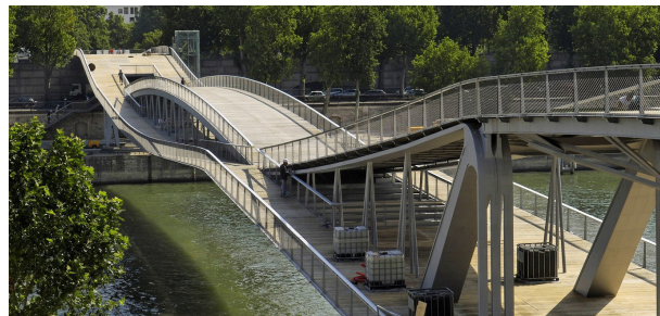
PASSERELLE SIMONE DE BEAUVOIR - FEICHTINGER
